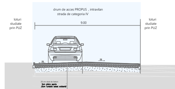
PROFIL TRANSVERSAL DRUM DE ACCES INTRAVILAN PROPUȘ
